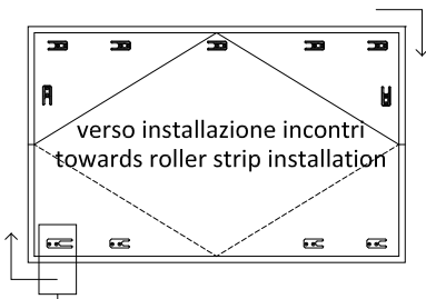
Riscontro anti falsa manovra Mishandling device strike
