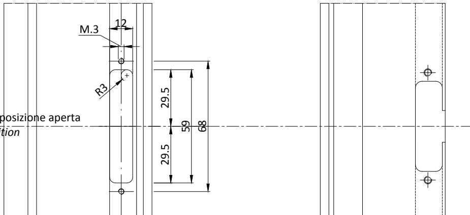
lavorazione applicazione nottolino Processing for plug installation
