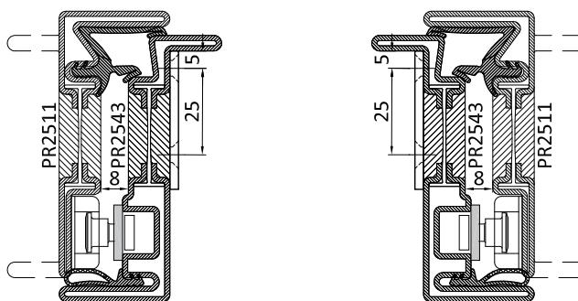
Sezione | Section B
