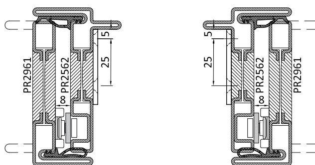
Sezione | Section A
