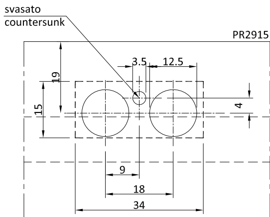
Particolare | Detail A
