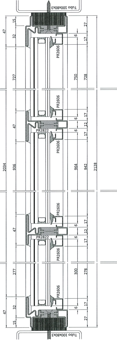
FINESTRA con FISSI OS2 65 apertura interna
