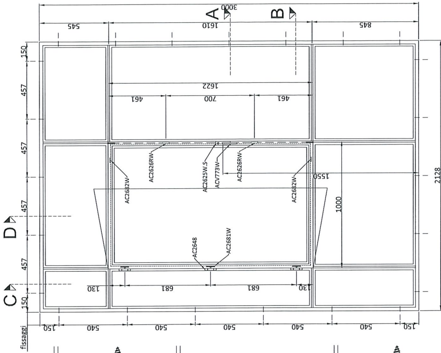
FINESTRA con FISSI OS2 65 apertura interna
