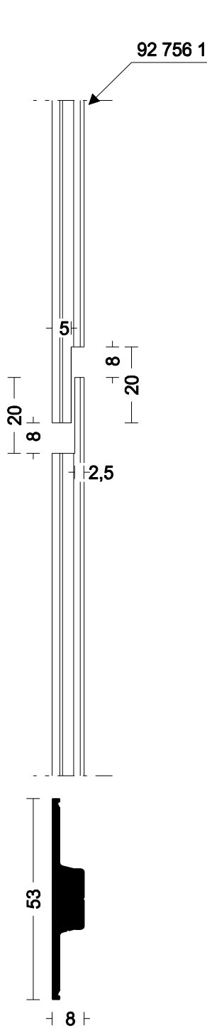
Ausklinkung SG-Andruckprofil
