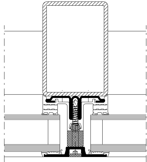
Anwendungsbeispiel 3-Ebenenendichtung Pfosten mit SG Andruckprofil mit sichtbarer, verdeckter Verschraubung
