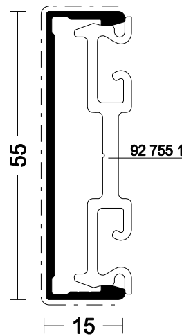
ALU 92 760 1 *
