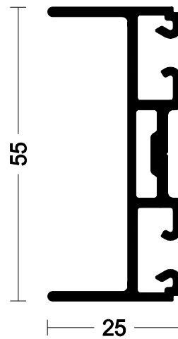
ALU 92 757 1 *
