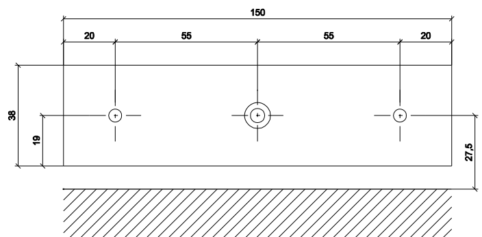
Sägebeilage 92-970301
