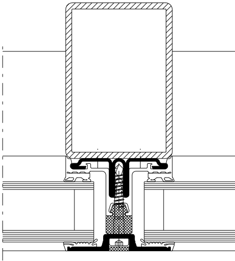
Anwendungsbeispiel 2-Ebenenendichtung Pfosten mit SG-Andruckprofil mit sichtbarer, verdeckter Verschraubung
