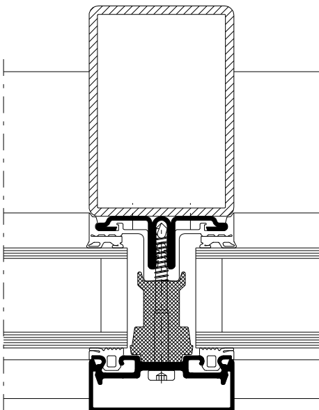
Anwendungsbeispiel 2-Ebenenendichtung mit Kreuzschaumkeder, Pfosten mit Alu Andruckprofil mit nicht sichtbarer Verschraubung
