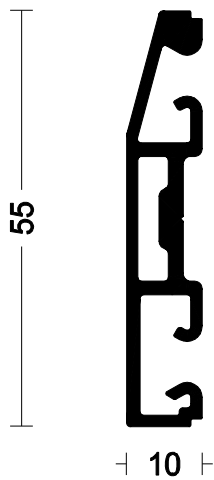
ALU 92 759 1 *
