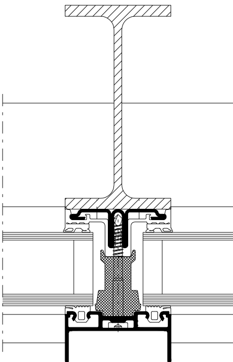
Anwendungsbeispiel 2-Ebenenendichtung mit Kreuzschaumkeder, Pfosten mit Alu Andruckprofil mit nicht sichtbarer Verschraubung
