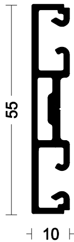
ALU 92 758 1 *
