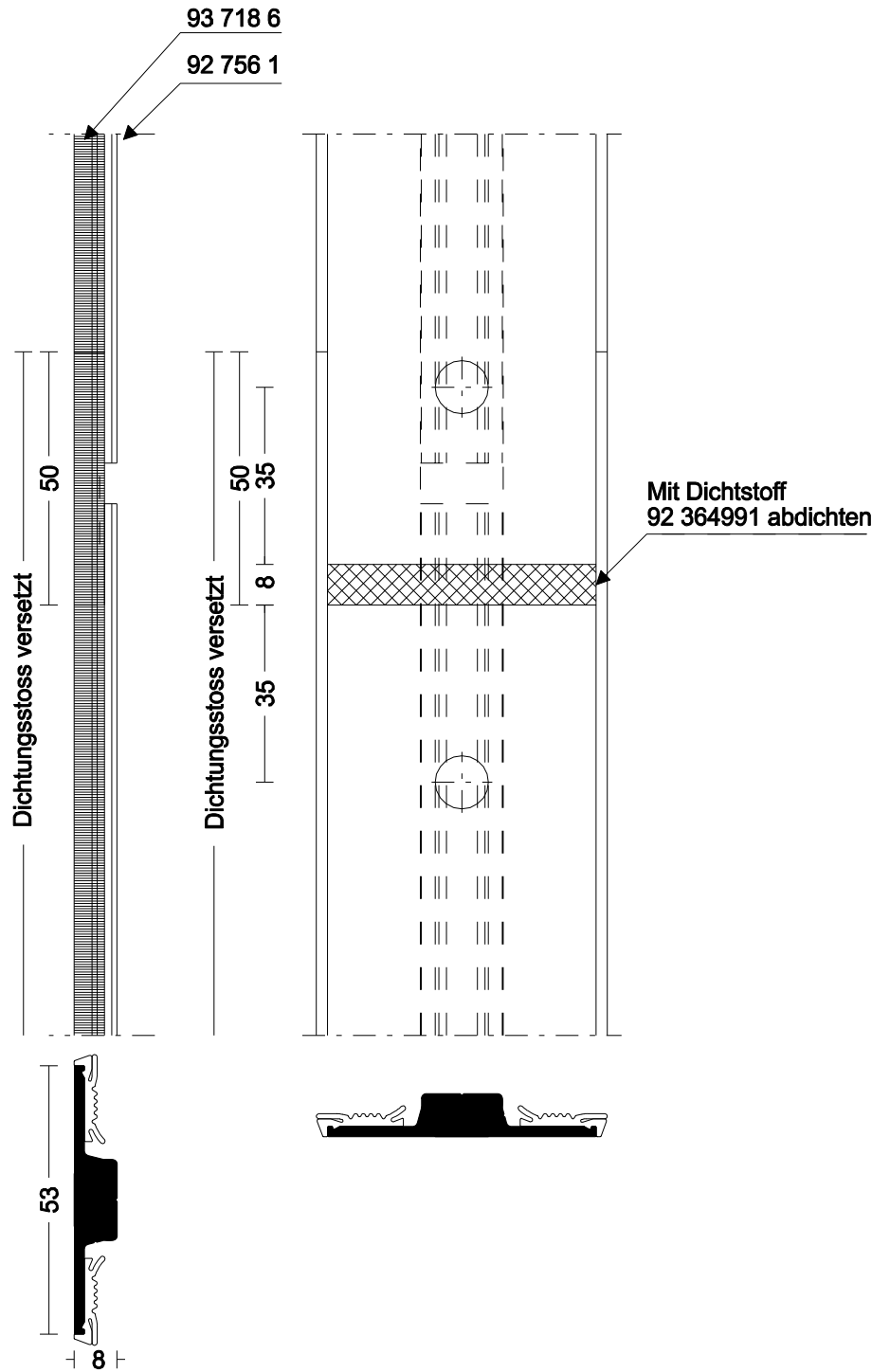
Vertikalstoss SG-Andruckprofil mit überlappender Dichtung
