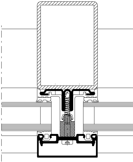
Anwendungsbeispiel 2-Ebenenendichtung Pfosten mit Alu Andruckprofil mit nicht sichtbarer Verschraubung
