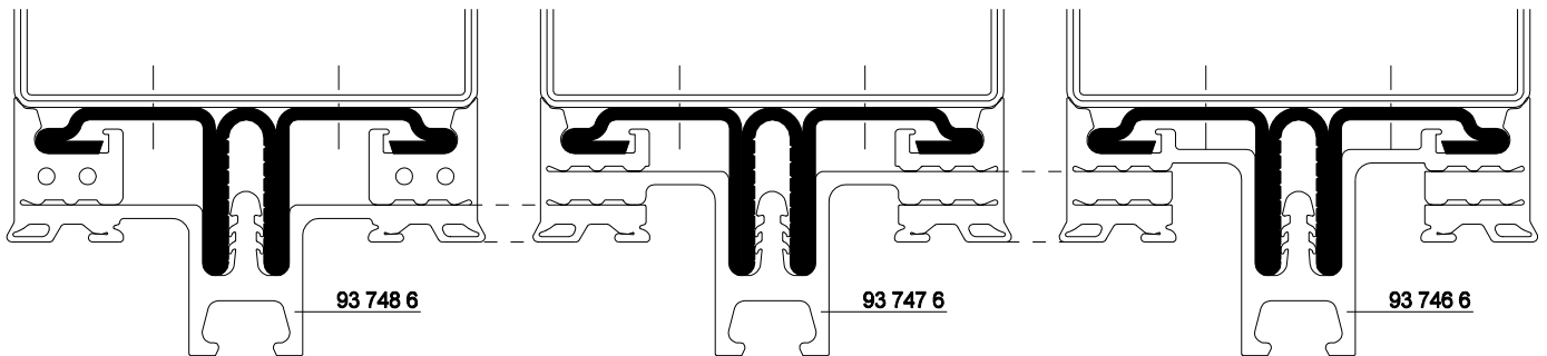
Detail E (siehe Seite 2.0.16) Detail J
