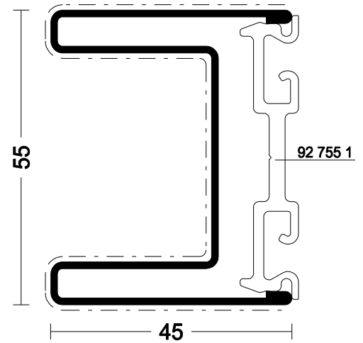
CRNI 92 762 4 *
