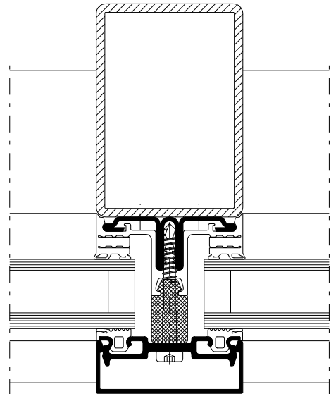
Anwendungsbeispiel 3-Ebenenendichtung Pfosten mit Alu Andruckprofil mit nicht sichtbarer Verschraubung
