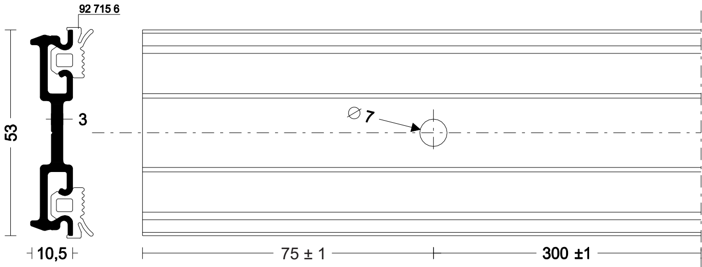
ALU 92 755 1 *
