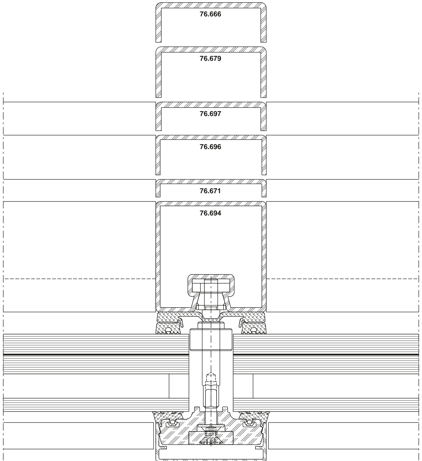
VISS Fassade Pfofen-Detail Ansichtsbreite 50 mm
